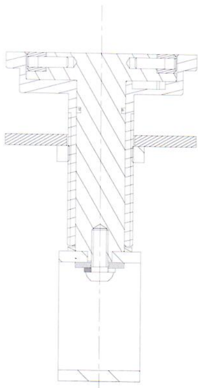
SEZIONE B-B
