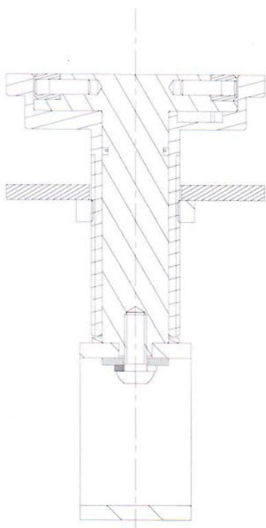
SEZIONE B-B
