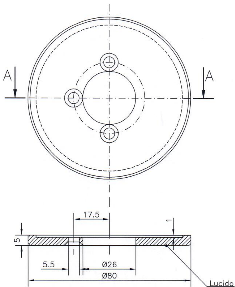
Sezione A:A
